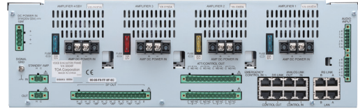
Mặt sau VX-3004F (Với mô-đun tăng âm cài sẵn)
