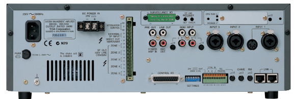
Mặt sau của VM-2120 / VM-2240
